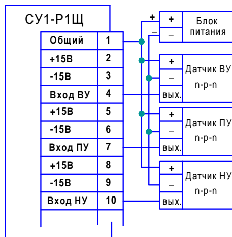
Рис. Б5. Схема подключения бесконтактных выключателей типа п-р-п при их питании от внешнего источника
