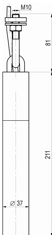
Габаритный чертёж
