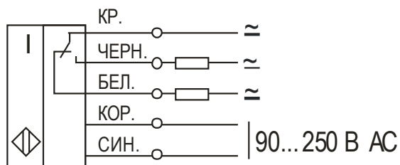
Схема подключения
