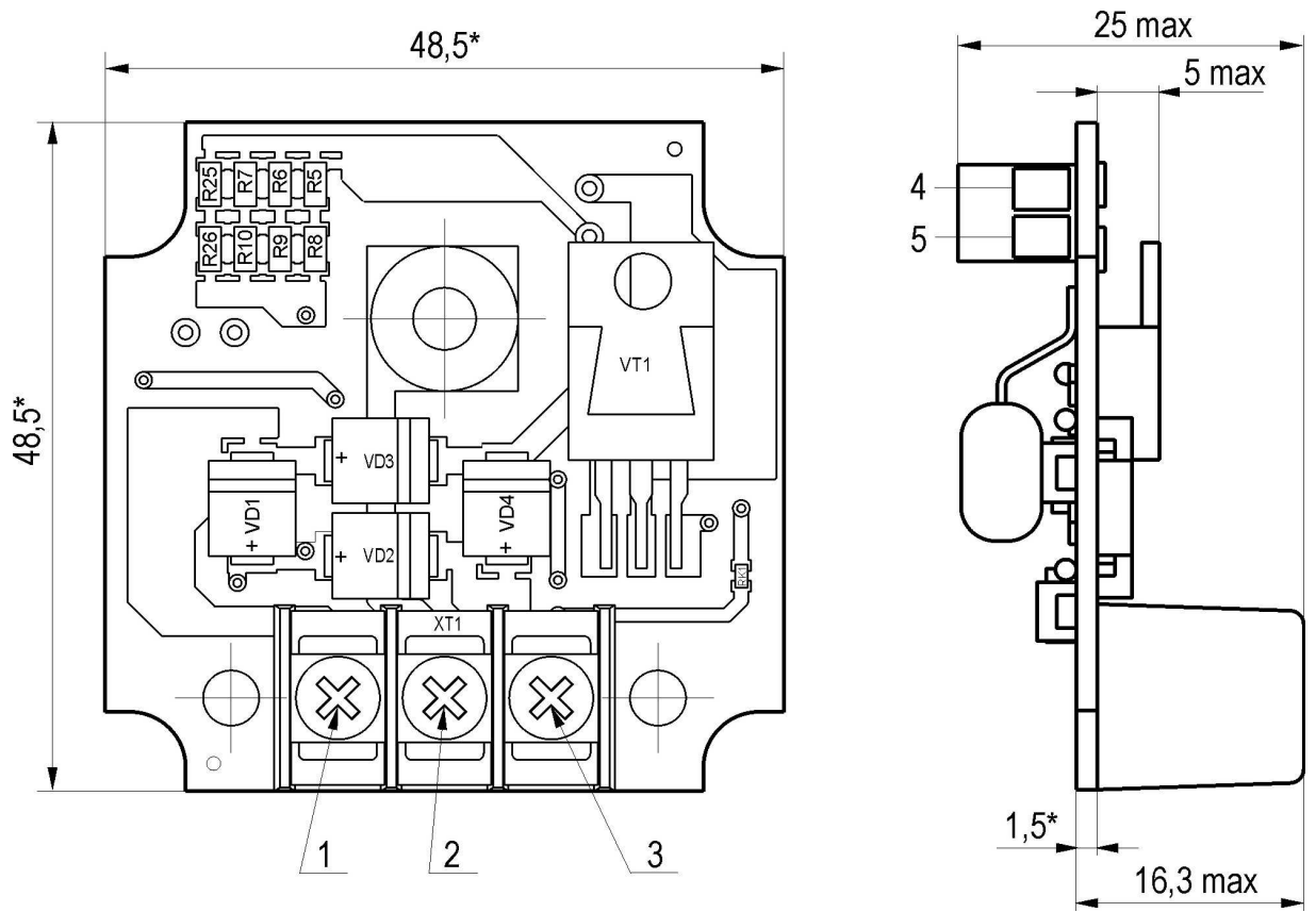
Рисунок 2. Габаритный чертёж Блока Удержания.
